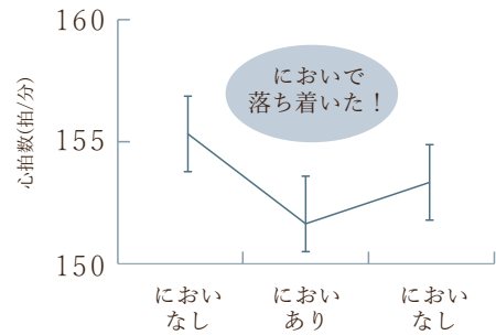
α-ピネンのにおいに対する乳児の心拍数の変化 (N=30, 平均値±標準誤差)
